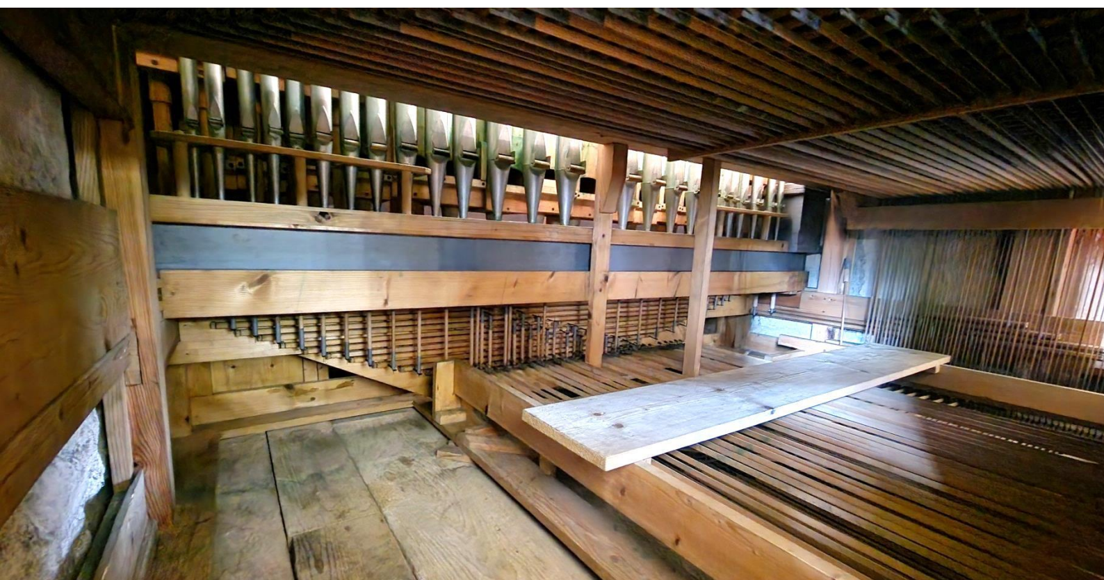
- Pohľad na pedálovú vzdušnicu, manuálovú traktúru a rozvodovú dosku pedálovej traktúry
